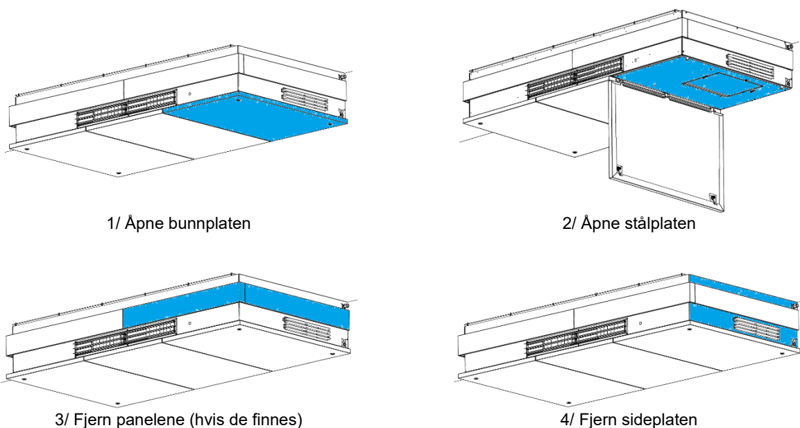
Figur 3: Få tilgang til tilkoblingene
