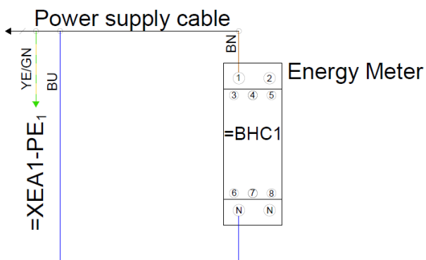
Figur 15: Enfasert energimåler
