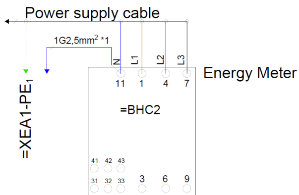
Figur 16: Trefase energimåler
