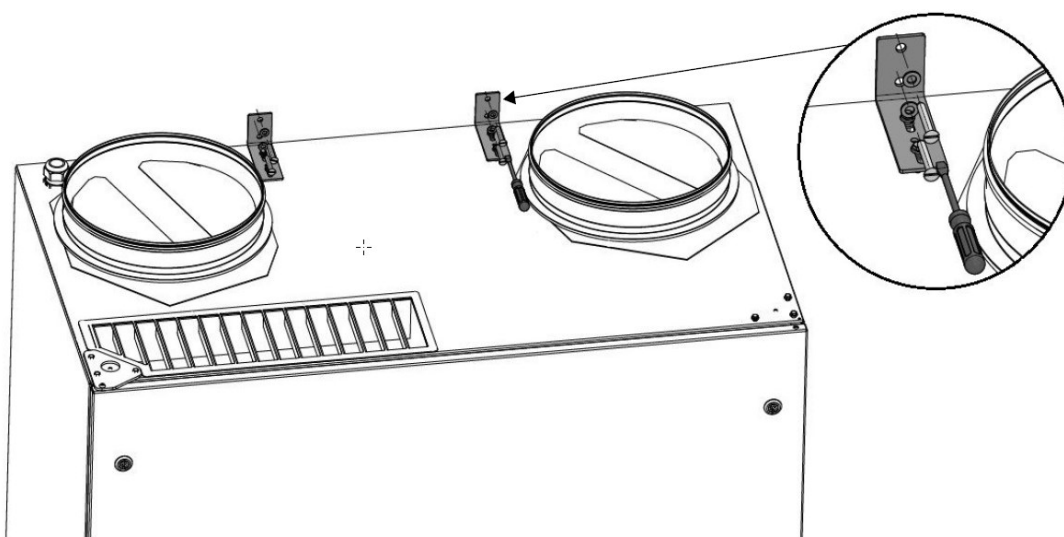
Figur 28: Fest braketten på toppen av anlegget til veggen
