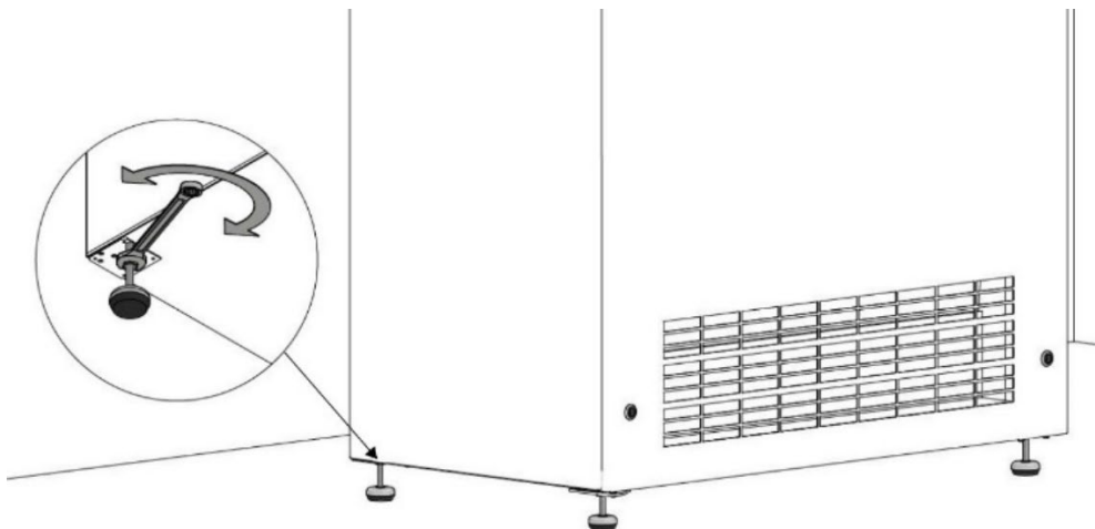
Figur 27: Juster føttene slik at anlegget blir i vater
