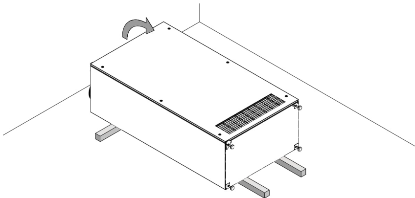
Figur 25: Plasser lekter/treblokker før du løfter anlegget
