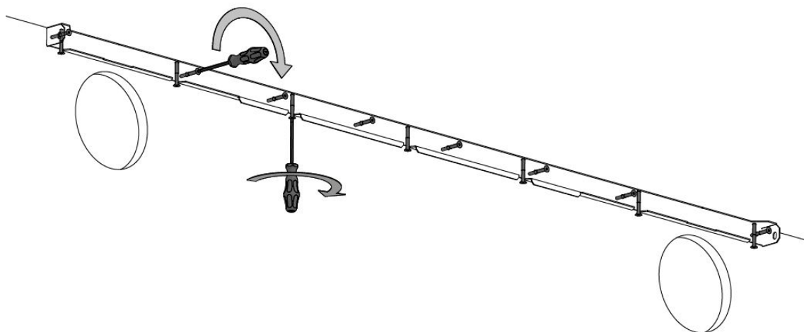
Figur 17: Monter beslaget
